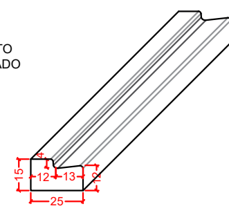
MEIO-FIO REBAIXADO TIPO 7 ESCALA 1 : 25
