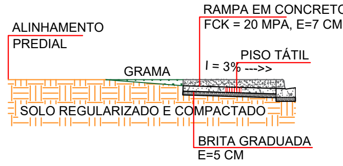
CORTE RAMPA DE ACESSIBILIDADE ESCALA 1 : 50
