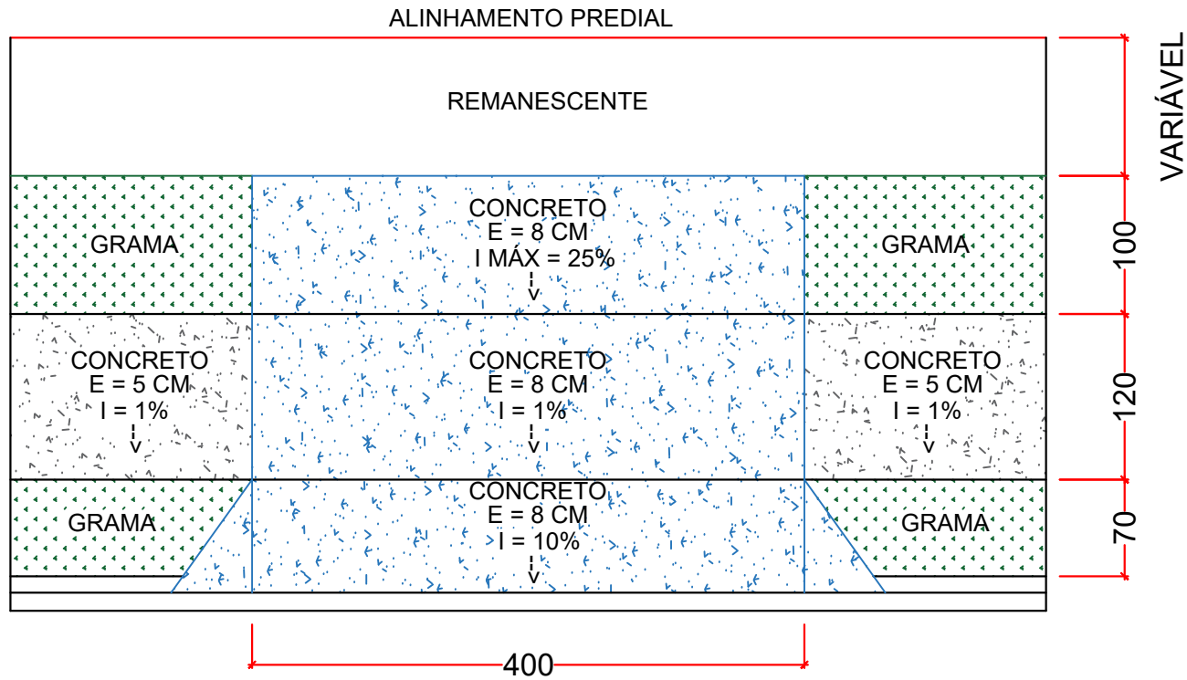
RAMPA PARA ACESSO DE VEÍCULOS ESCALA 1 : 50
