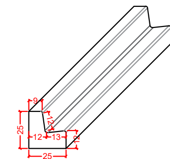
MEIO-FIO TIPO 2 ESCALA 1:25
