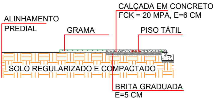
CORTE CALÇADA ESCALA 1 : 50
