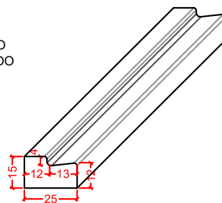
MEIO-FIO REBAIXADO TIPO 7 ESCALA 1:25
