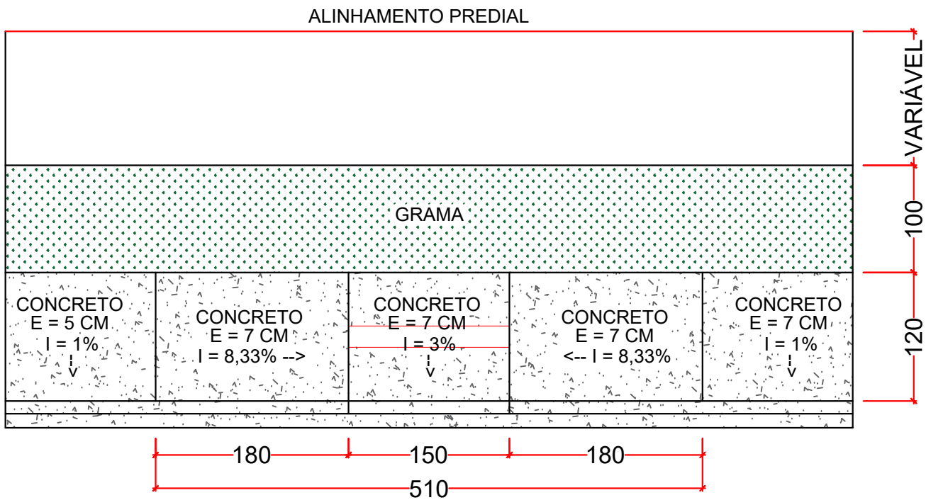
RAMPA DE ACESSIBILIDADE ESCALA 1 : 50
