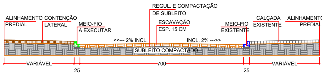
CORTE A-A'
