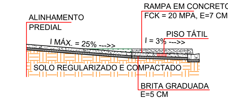
CORTE RAMPA PARA ACESSO DE VEÍCULOS ESCALA 1 : 50
