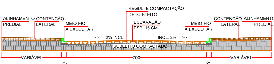
Perfil de corte
