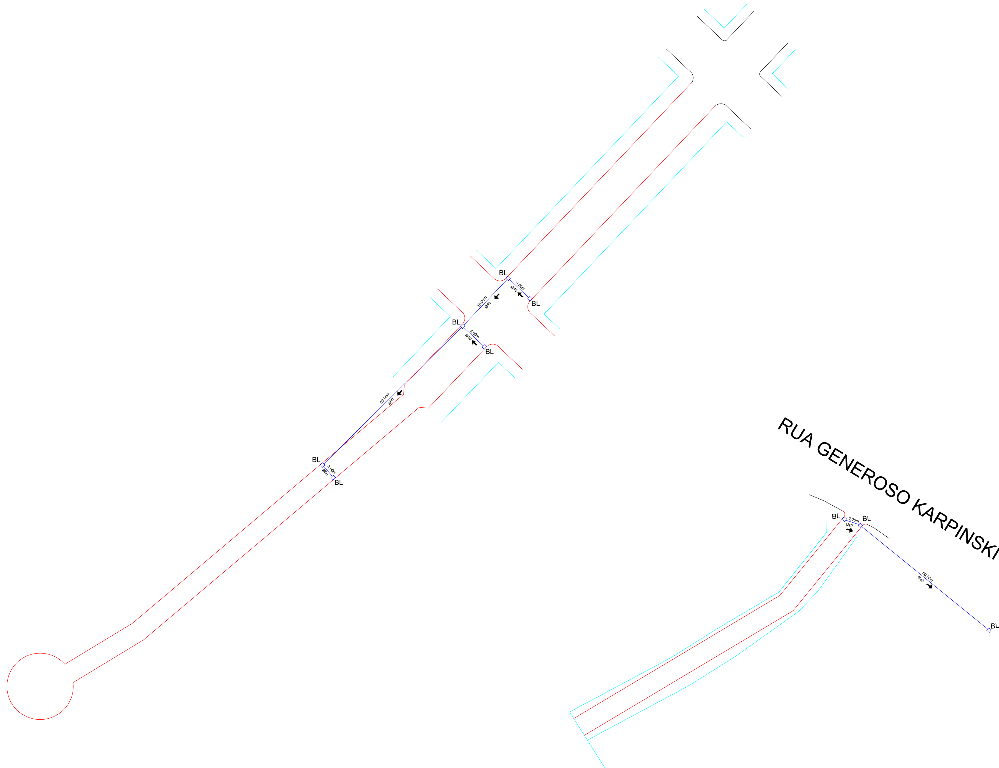
PLANTA DA REDE DE CAPTAÇÃO DE ÁGUAS PLUVIAIS Escala: 1/500
