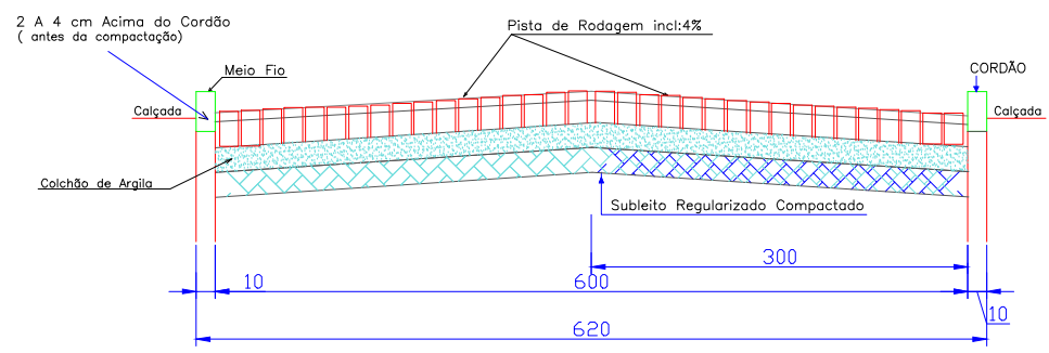
CORTE TRANSVERSAL S/ ESC.
