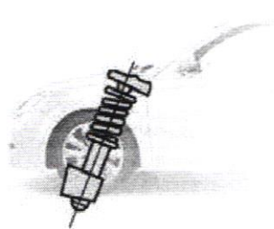
Ângulo de caster positivo
