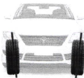
Cambagem positiva
