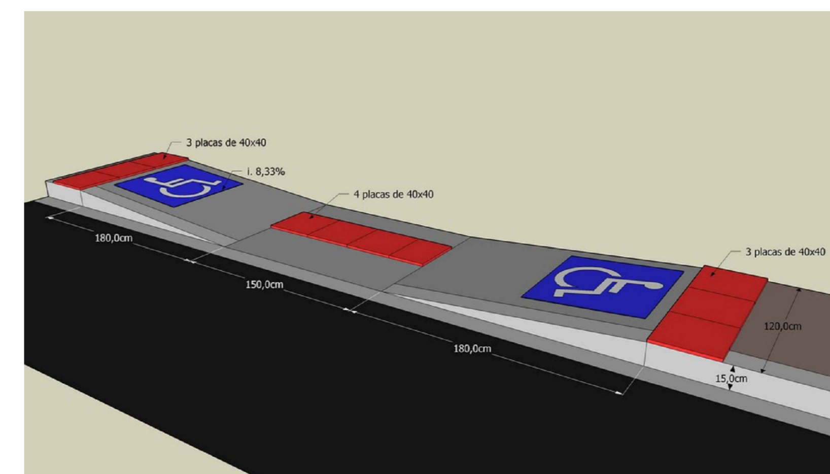
DETALHE DA RAMPA SEM ESCALA
