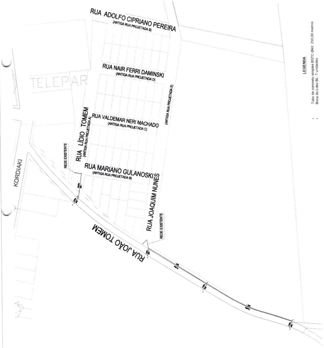
PLANTA DA REDE DE CAPTAÇÃO DE ÁGUAS PLUVIAIS Escala: 1/750
